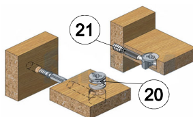
Эксцентриковая стяжка
