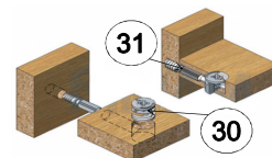
Эксцентриковая стяжка
