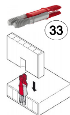
Однокомпонентная стяжка
