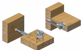
Эксцентриковая стяжка
