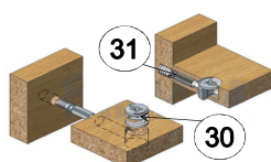
Эксцентриковая стяжка
