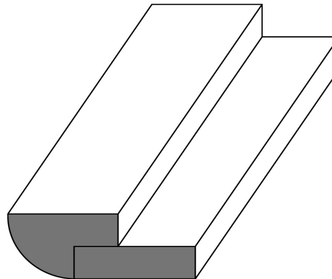
Карниз №1 Правый Габаритные размеры (ШхГ), мм: 3092 x 508
