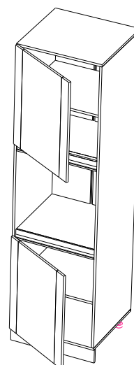
ПГ-60 600x586x2166 Ш Г В
