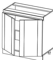
С-80 800x450x820 Ш Г В
