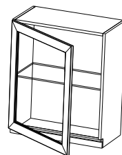
ШСТ-60 600x320x720 Ш Г В
