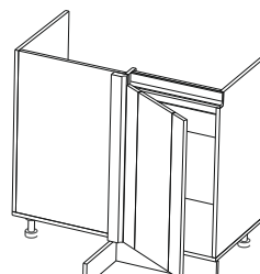
СМУ-100п 900x450x820 Ш Г В
