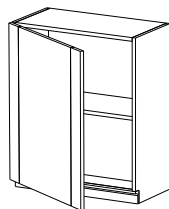
ШГ-60 600x320x720 Ш Г В
