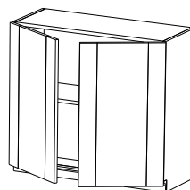
ШГ-80 800x320x720 Ш Г В
