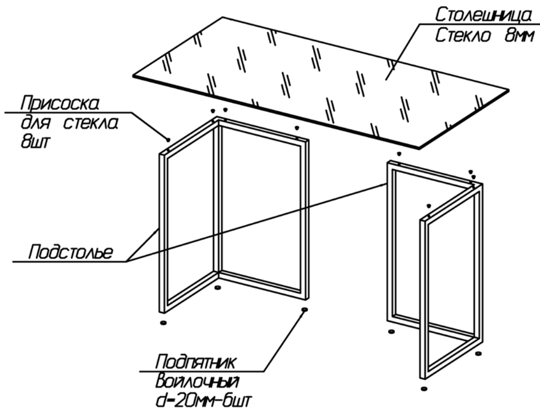
Рис. 2 Схема сборки стола (материал столешницы: стекло 8мм)
