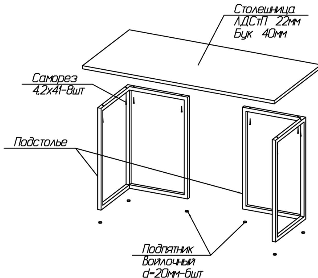
Рис. 1 Схема сборки стола (материал столешницы: ЛДСП 22мм/Бук 40мм)
