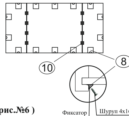
СХЕМА РАСПОЛОЖЕНИЯ ФИКСАТОРОВ
